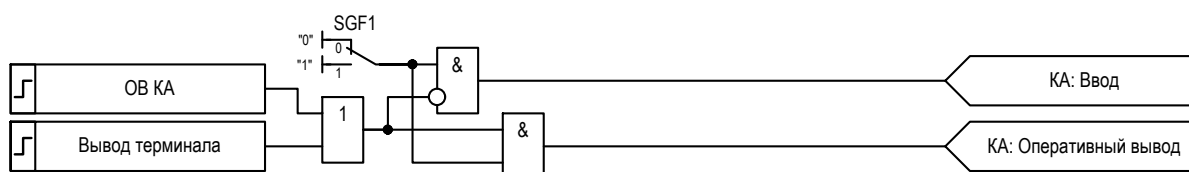
Рисунок 2.32 – Логика управления режимами функционального блока «КА»
