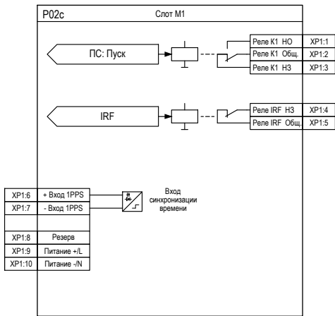
Рисунок Е.1 – Подключение дискретных входов и выходов к внутренним сигналам алгоритмов для блока в слоте M1
